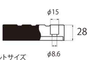
穴径断面図
