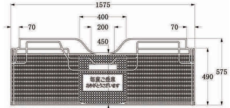
参考肉厚:4mm(外周縁部5mm) MT-14CBR クラウンコンフォート用 リヤー
