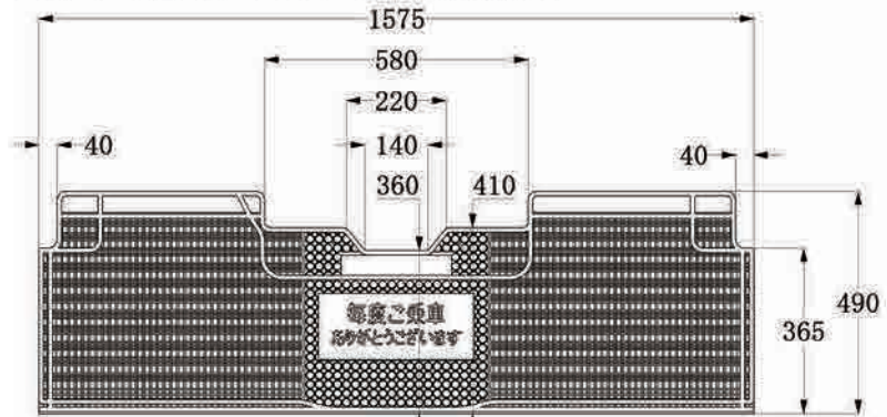
参考肉厚:4mm(外周縁部5mm) MT-16CBR マークII コンフォート用 リヤー
