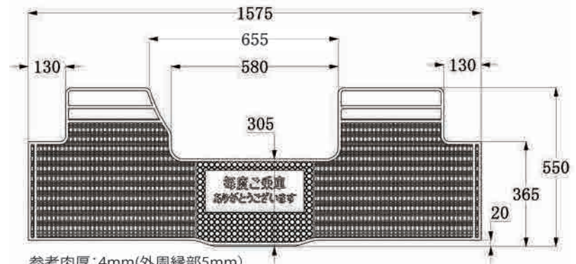
参考肉厚:4mm(外周縁部5mm) MT-15CBR ニッサン クルー用 リヤー
