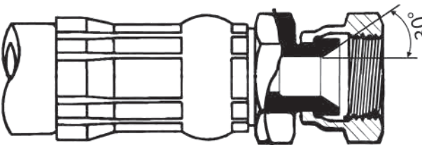
洲本タイプ以外 【1004管用めねじユニオン(めすシート)タイプ】
