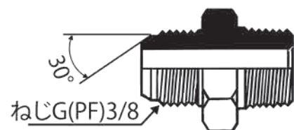
【1013管用アダプター(おすシート)タイプ】
