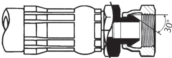
洲本タイプ以外 【1004管用めねじユニオン(めすシート)タイプ】
