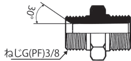
【1013管用アダプター(おすシート)タイプ】
