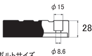
穴径断面図
