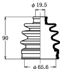
材質 ゴム
